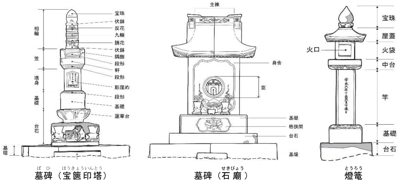
図 石造物 各部位名称
